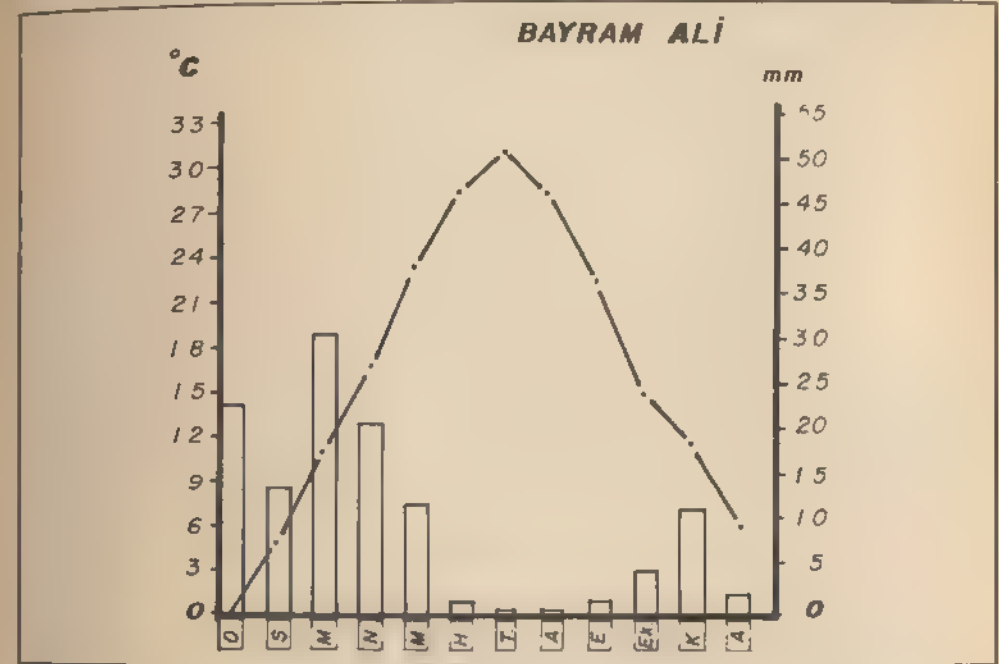
Şekil 6 - Bayram Ali'nin iklim diyagramı. Sıcaklık kesik çizgi ile, yağış sütunlarla gösterilmiştir
